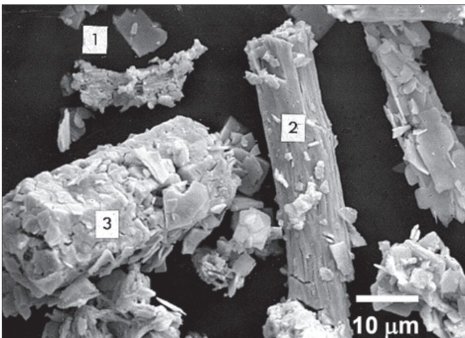
Elektronenmikroskopische Aufnahme von MOX (Mischoxid) Brennstoff, der 1994 auf dem Flughafen München beschlagnahmt wurde. Die Plättchen (1) und das zylindrische Partikel (2) bestehen aus \text{PuO}_2 , das größere sechseckige Partikel (3) aus \text{U}_3\text{O}_8 (© European Communities).
