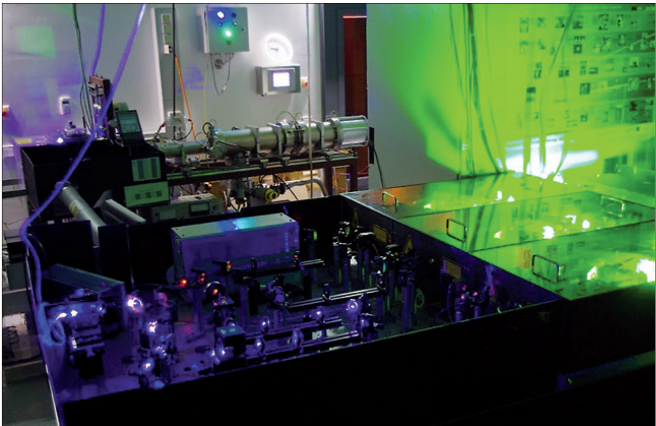
Das Foto zeigt im Vordergrund die Laserapparatur für die Resonanzionisations-Massenspektrometrie (RIMS), die am Institut für Kernchemie der Universität Mainz zum Ultrapurennachweis von Plutonium, Neptunium und Technetium eingesetzt wird. Mit dem von einem Nd:YAG-Laser erzeugten grünen Laserlicht werden drei Ti:Saphir-Laser gepumpt. Das blaue Laserlicht entsteht durch Frequenzverdopplung des von einem der Ti:Saphir-Laser abgegebenen fundamentalen Laserlichtes. Im Hintergrund ist das Flugzeit-Massenspektrometer (TOF-MS) zum Nachweis der durch die Laserstrahlung selektiv ionisierten Radioisotope zu sehen. (© Nils Stöbener, Institut für Kernchemie, Universität Mainz)
