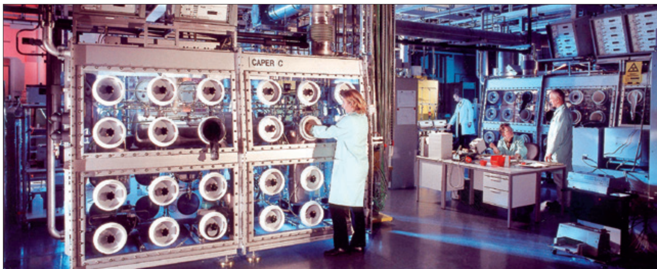
Blick in das Tritiumlabor des KIT (© KIT 2002, Martin Lober, Markus Breig)
