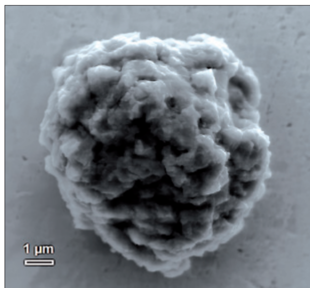
Sternenstaub von Roten Riesen – Siliziumkarbid-Korn aus dem Meteoriten Murchison. (© J. Huth, S. Merchel, MPI Mainz)
