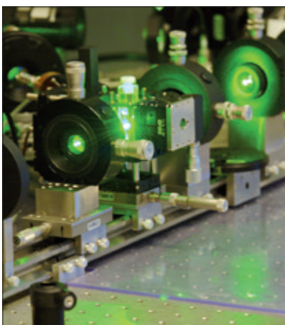
Links: Aufbau zur Aufklärung der chemischen Form gelöster Actinidionen mittels Laserspektroskopie (© KIT, Coerten); rechts: Experimente zur Radionuklidmigration im Grimsel Felslabor, Schweiz (© COMET, Photoshopping, GmbH, Weisslingen)
