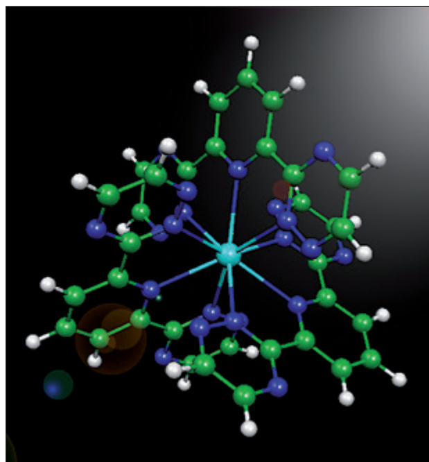
Komplex des dreiwertigen Americiumions mit drei Bis-triazinylpyridin Molekülen. Dabei handelt es sich um ein vielversprechendes Extraktionsreagenz für die Actiniden/Lanthaniden-trennung. (© KIT)
